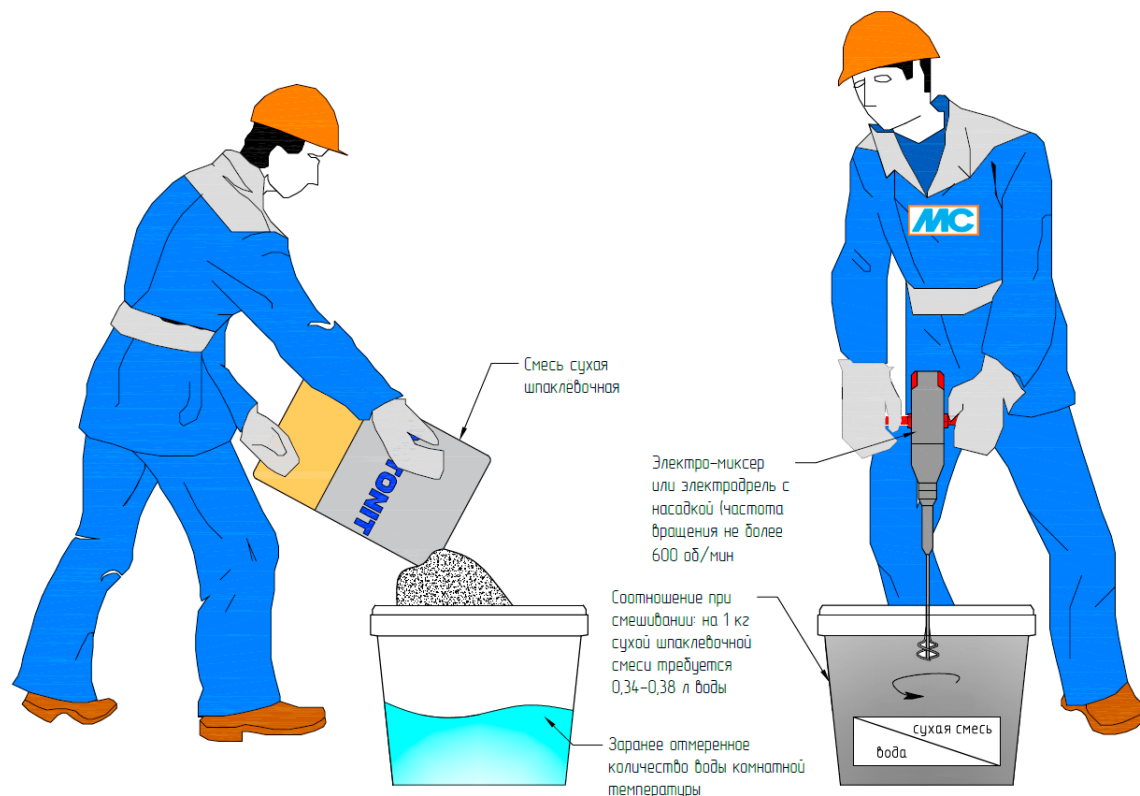
Рис. 28. Организация работ по затворению сухой шпаклевочной смеси
