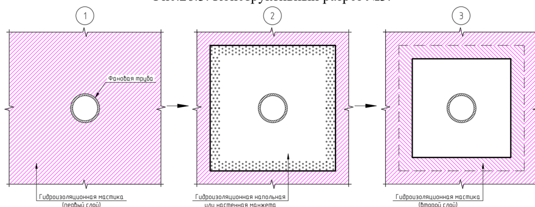
Рис.26.3. Конструктивный разрез №3.
